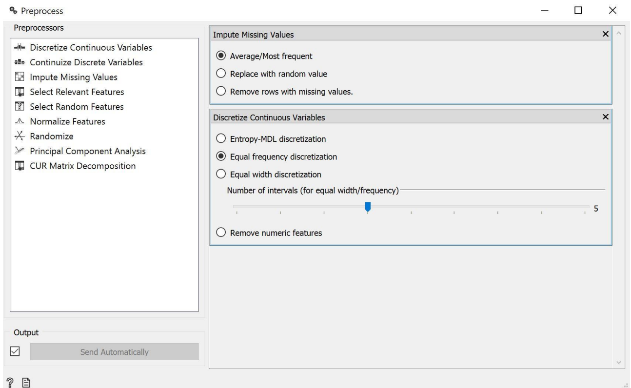
Εικόνα 14: Data preprocessing
