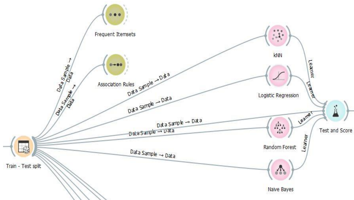
Εικόνα 22: Μοντέλα πρόβλεψης
