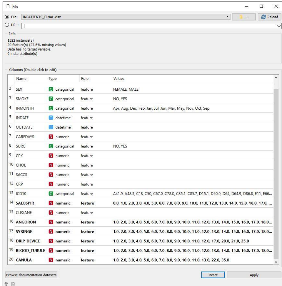
Εικόνα 6: File widget
