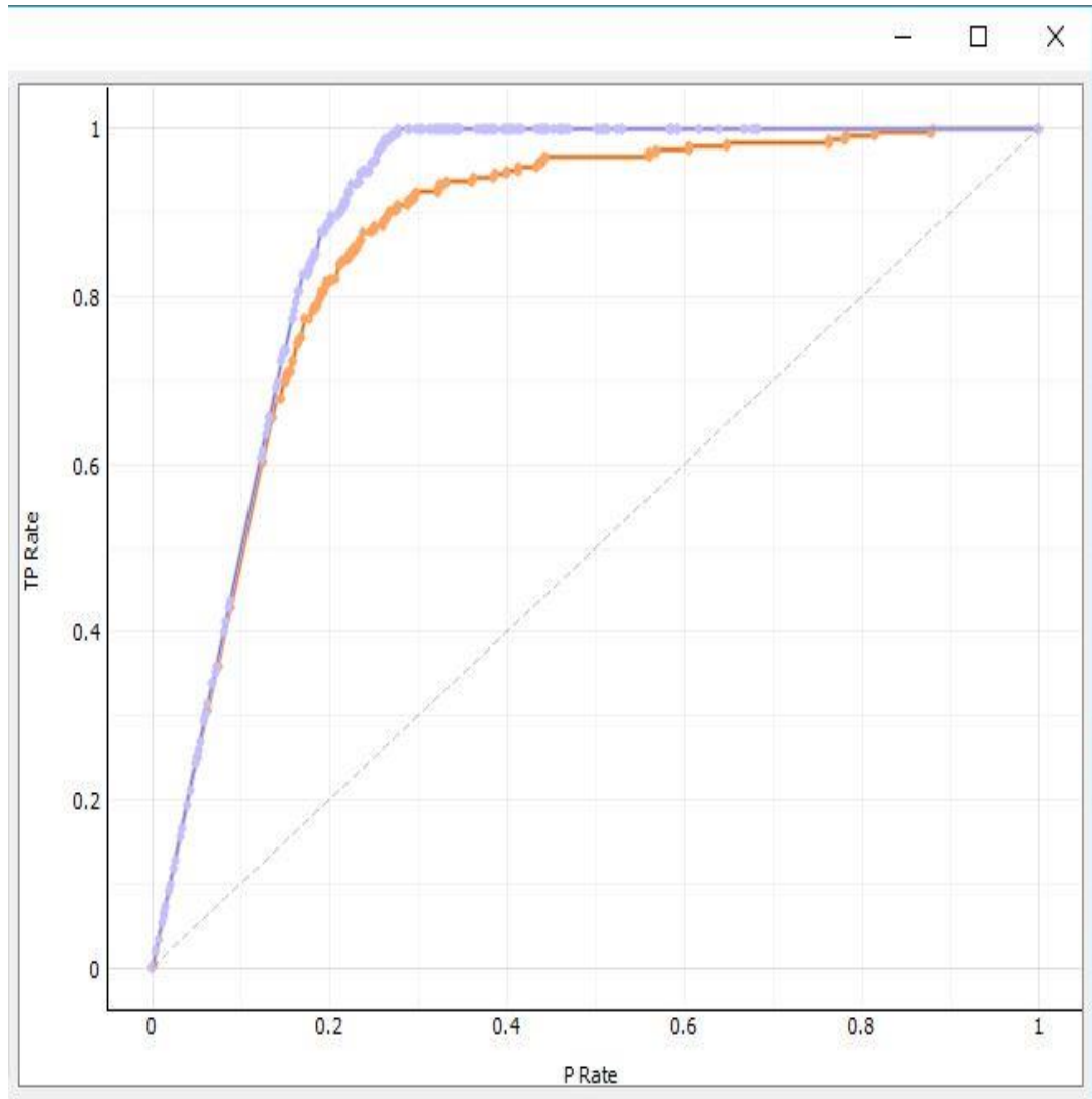
Εικόνα 27: Lift Curve
