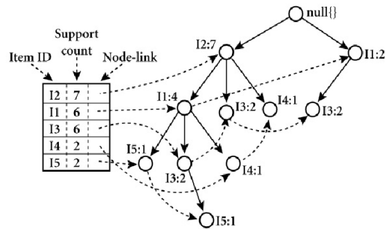
Εικόνα 5: FP-tree
