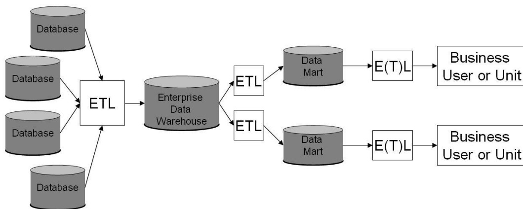
Εικόνα 2: Data Warehouse
