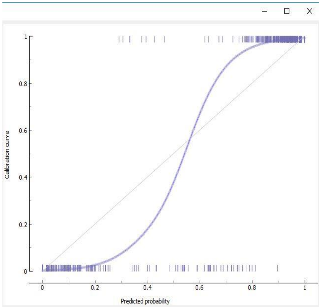
Εικόνα 26:Calibration Plot
