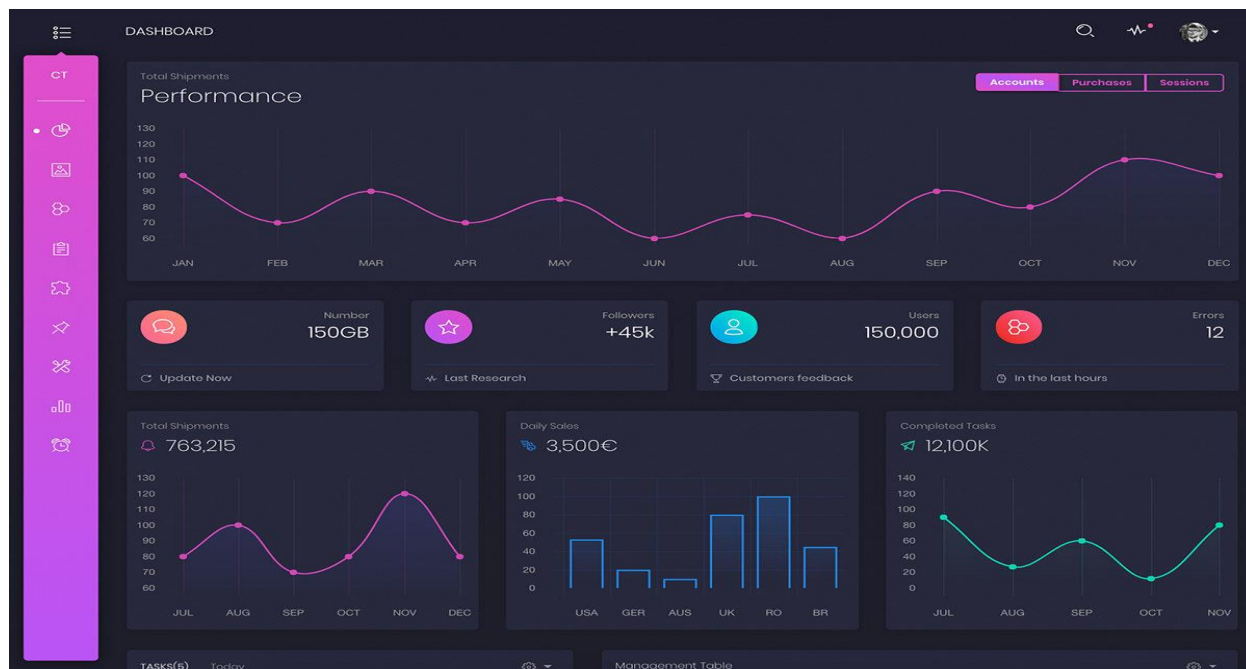
Εικόνα 3.9 Διεπαφή user
