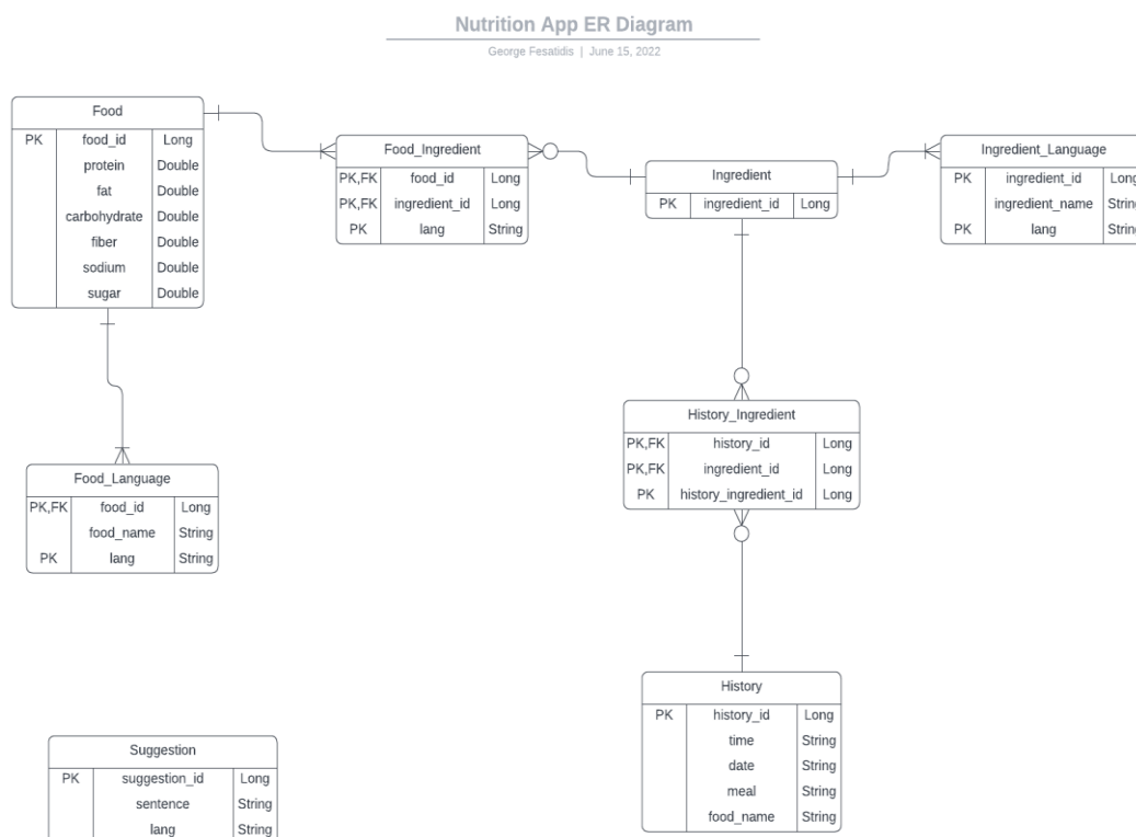
Εικόνα 23: Το Σχήμα Βάσης Δεδομένων της Διατροφικής Εφαρμογής
