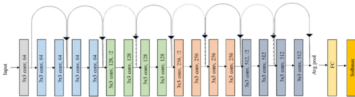
Εικόνα 4: Αρχιτεκτονική ResNet-18
